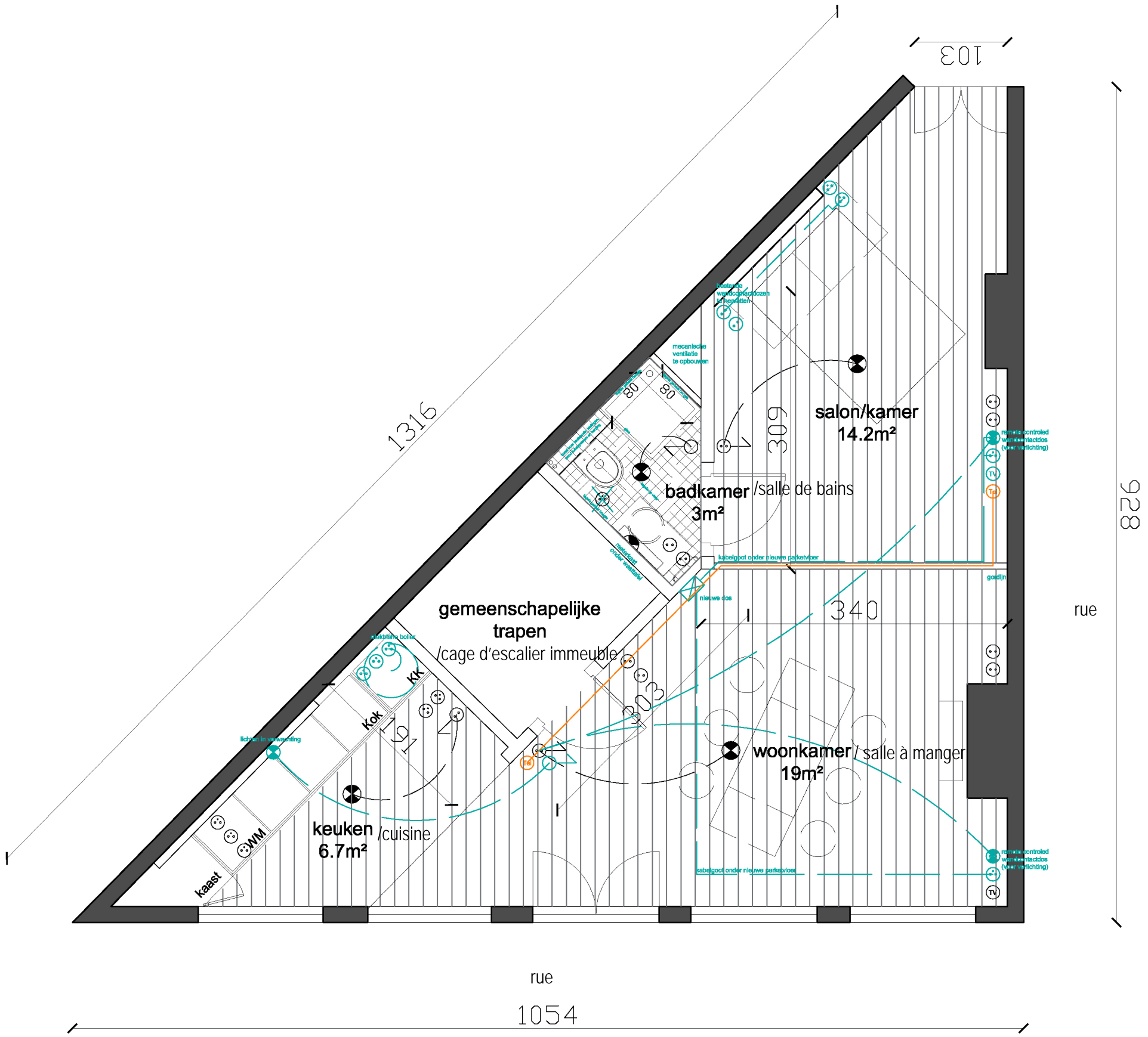
PLAN INTERIEUR APPARTEMENT
