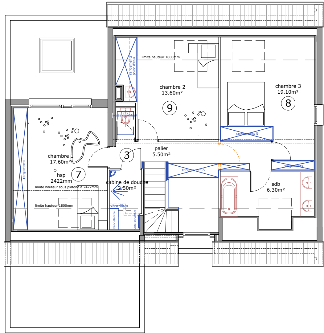
Plan Etage
